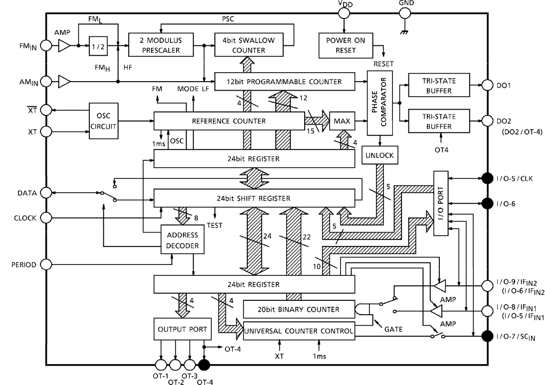
U260 / TC9257F
