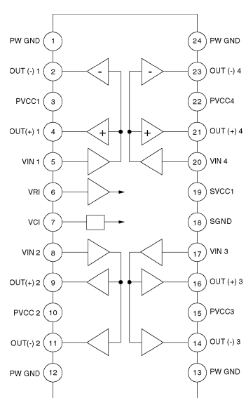
IC703 / TA2092N
