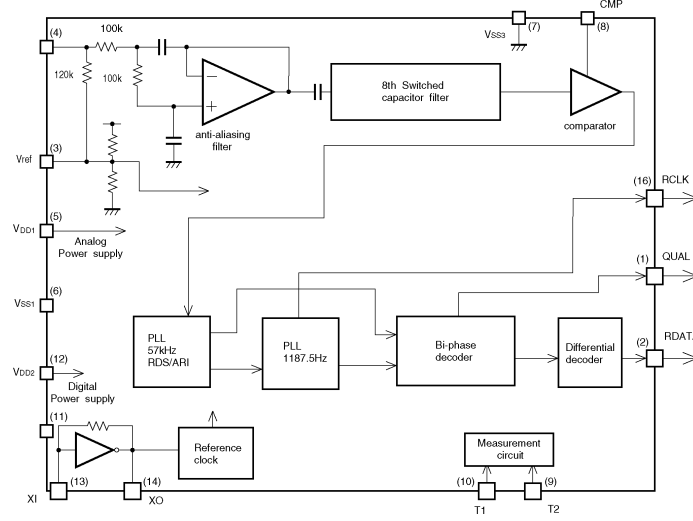
U250 / BU1924F
