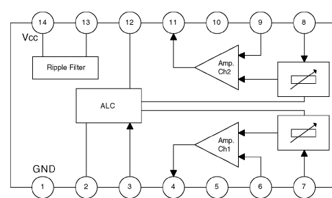
U301 / AN7312
