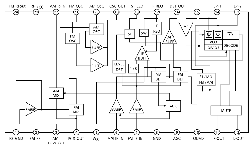
U201 / TA2104BN
