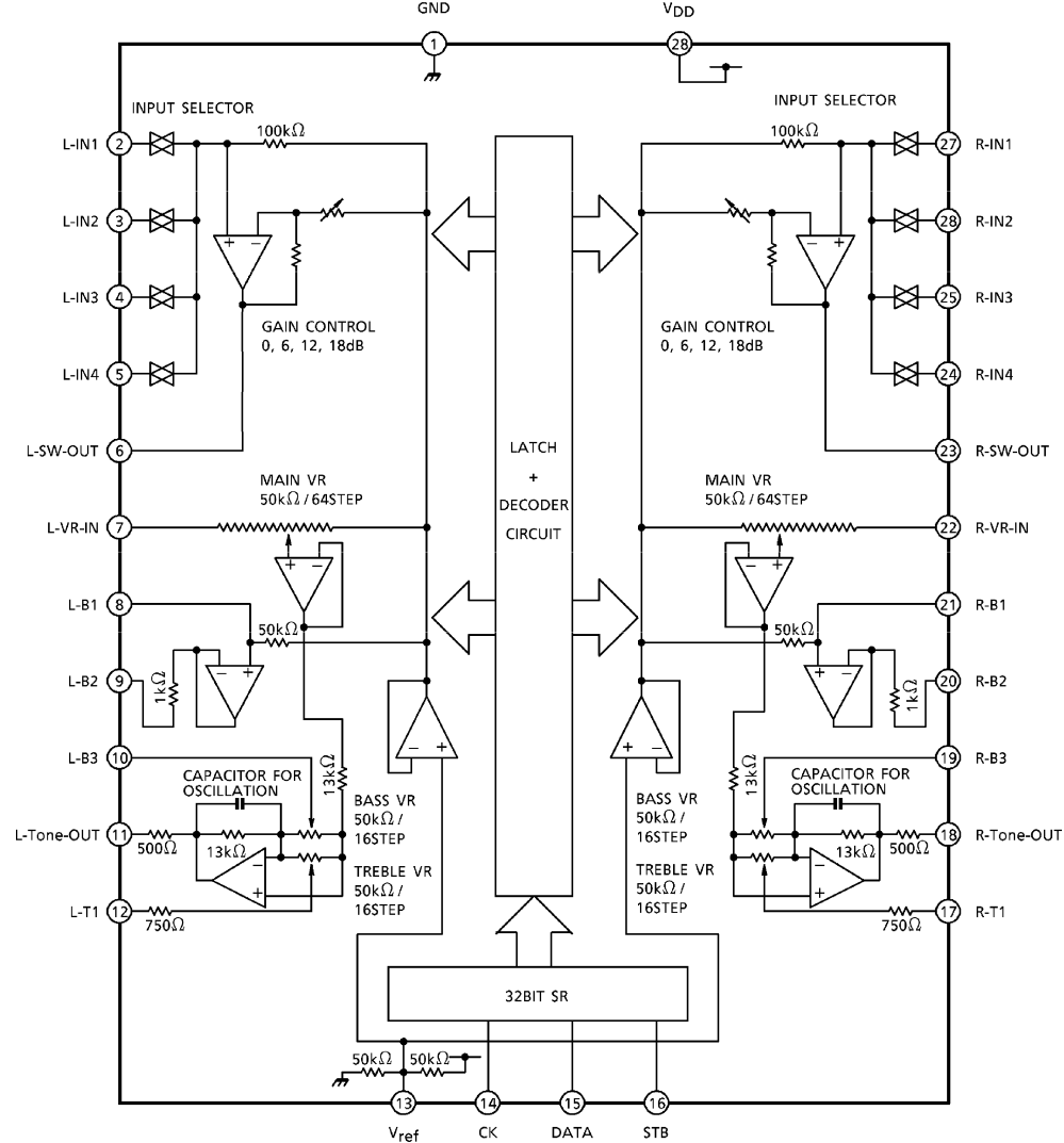
U601 / TC9422F
